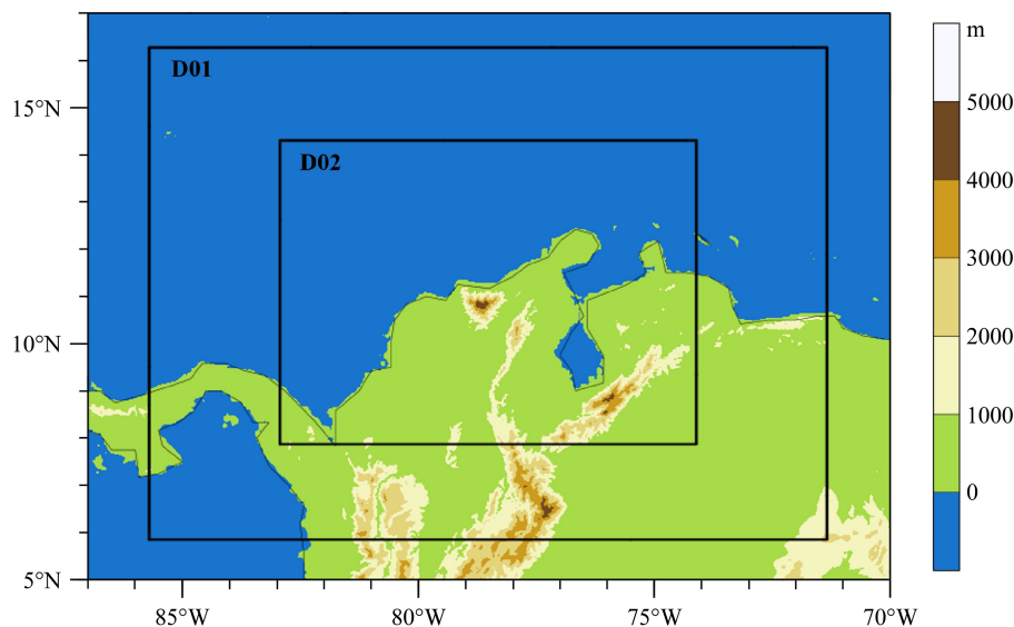
图 1 哥伦比亚北部研究区域高程图及 WRF 9 km 和 3 km 嵌套模拟方案示意图。
