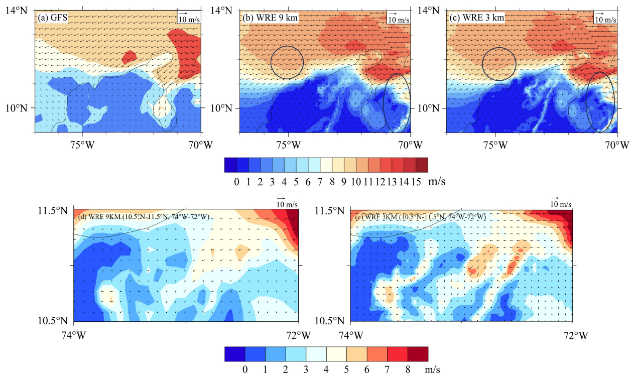
图 5 同图 4, 但为 2022 年 7 月 6~10 日。
