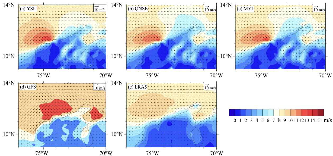
图 2 2022 年 1 月 6~10 日 (a) YSU、(b) QNSE、(c) MYJ 边界层参数化方案模拟数据、(d) GFS 预报数据 (起始时间为 2022 年 1 月 1 日) 与 (e) ERA5 再分析数据在哥伦比亚北部的平均风场空间分布。
