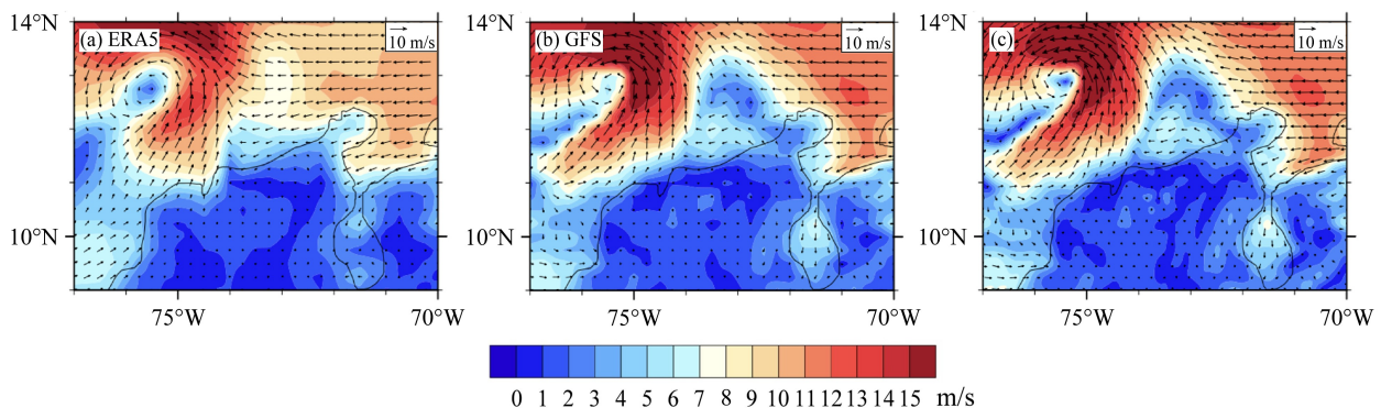
图 6 2022 年 10 月 8 日 00:00 哥伦比亚北部 (a) ERA5 再分析资料、(b) GFS 预报数据、(c) WRF 模拟数据飓风 Julia 风场分布。
