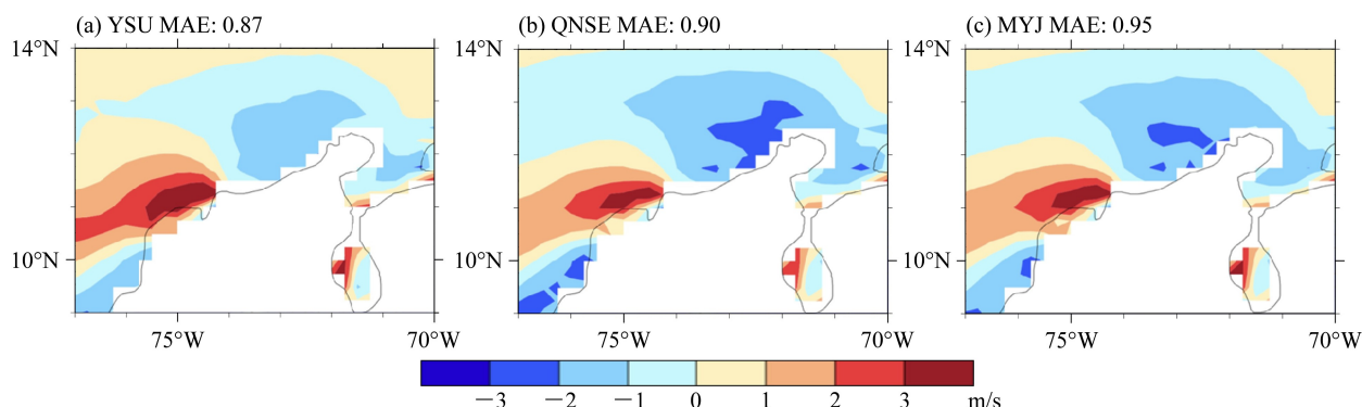
图 3 2022 年 1 月 6 日~10 日 (a) YSU、(b) QNSE、(c) MYJ 边界层参数化方案模拟的海上 10 m 风速在哥伦比亚北部相对于 ERA5 再分析数据的模式偏差空间分布 (起始时间为 2022 年 1 月 1 日)。
