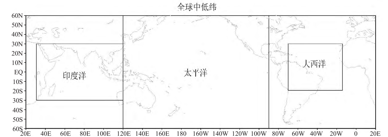
图 1 各研究区域的定义范围
