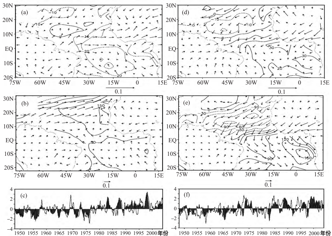
图4 同图2,但为大西洋的分析结果
