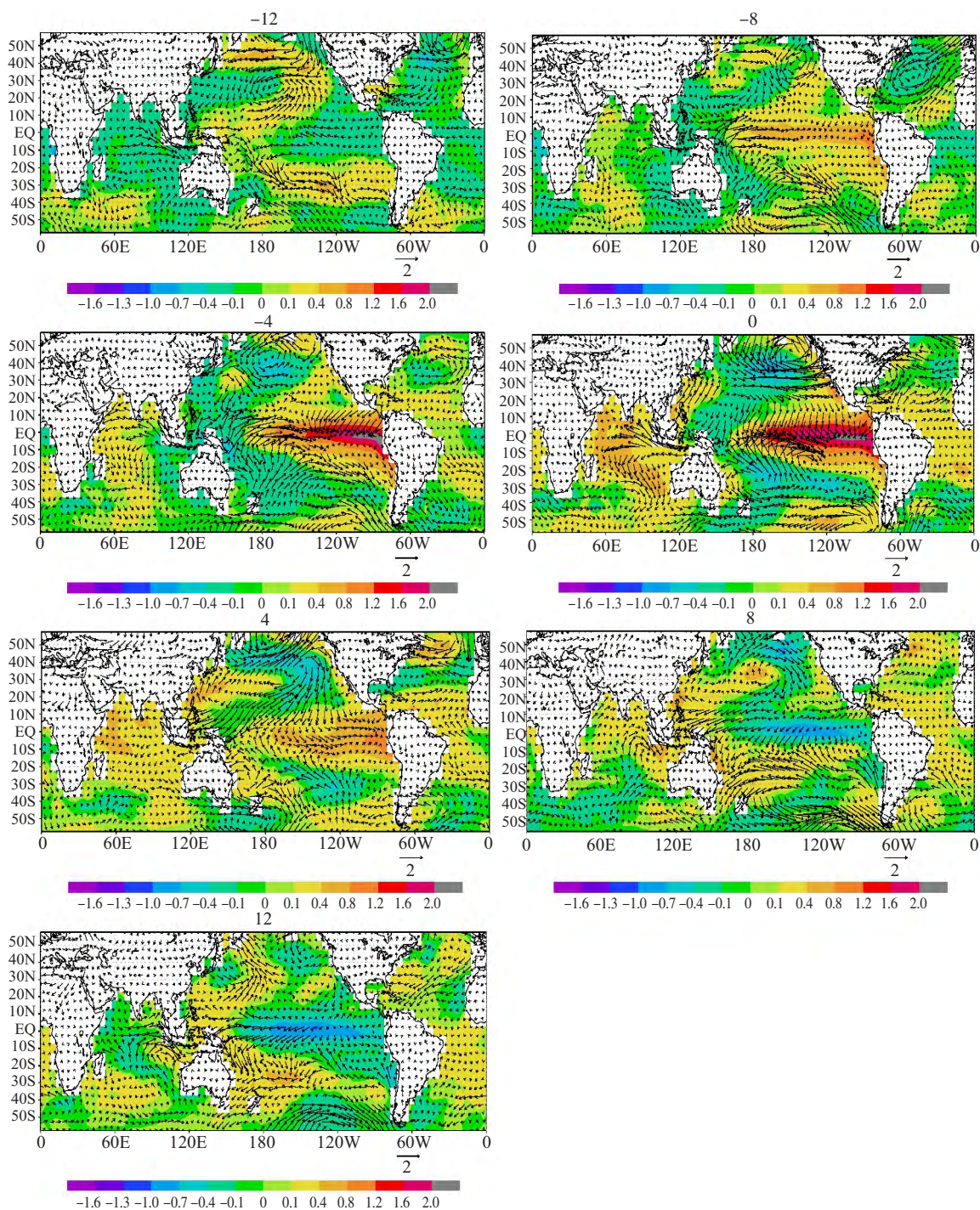
图7 7次正异常事件合成的超前滞后12个月的海温和风场异常演变
