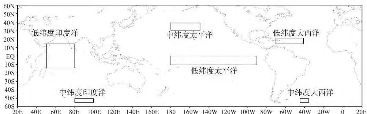
图 5 三大洋比较区域的范围定义
