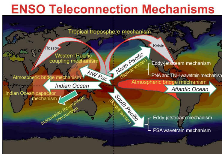
图 1 ENSO 影响全球天气气候的主要遥相关机制示意图。引自 Yang et al. (2018) 。
