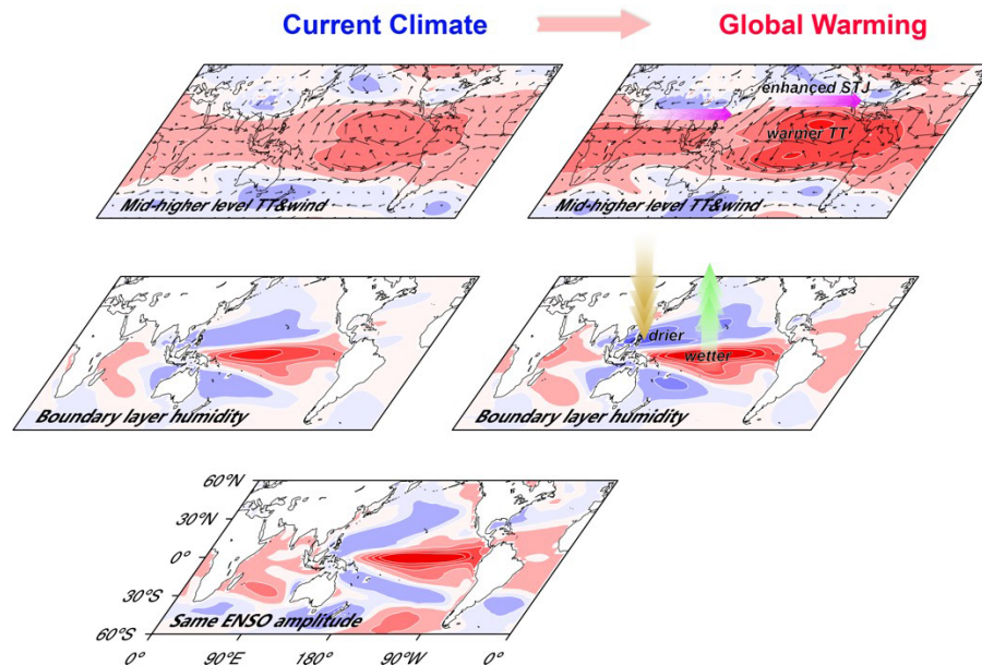
图4 全球变暖下 ENSO 热带遥相关变化示意图。修改自 Hu et al. (2021)。
