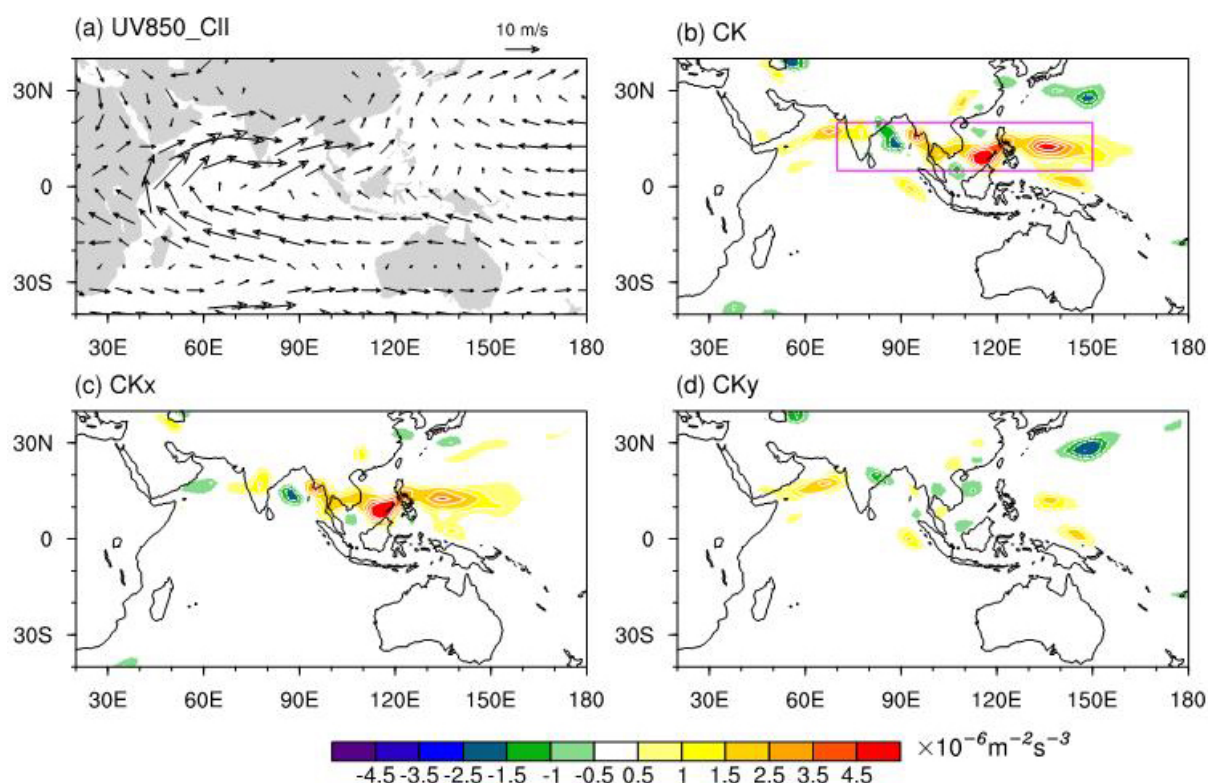
图2 El Niño 衰退年夏季西北太平洋背景场动能和扰动动能之间的转换。(a) 西北太平洋 850-hPa 气候态风场 (矢量, 单位: m/s), (b) 850-hPa 扰动场从背景场中获取的动能转换 (CK, 单位: \text{m}^2/\text{s}^3 ), (c) 和 (d) 分别为 CK 的纬向部分和经向部分 (单位: \text{m}^2/\text{s}^3 )。引自 Hu et al. (2019)
