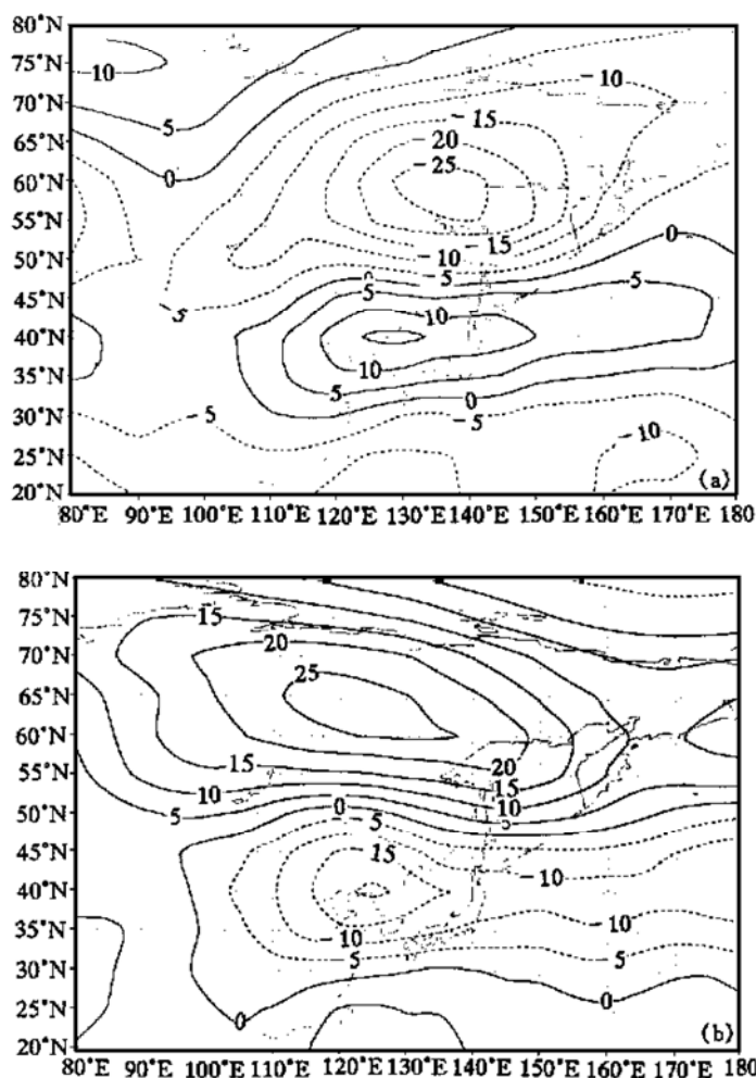
图2 由图1所示的高低 I_{EAP} 指数状况合成的东亚夏季500 hPa位势高度场距平
