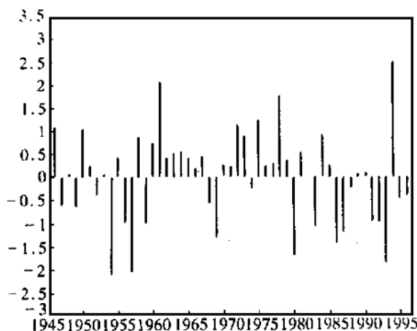
图1 东亚夏季风环流异常指数 I_{EAP} 的年际变化(1946~1996年)
